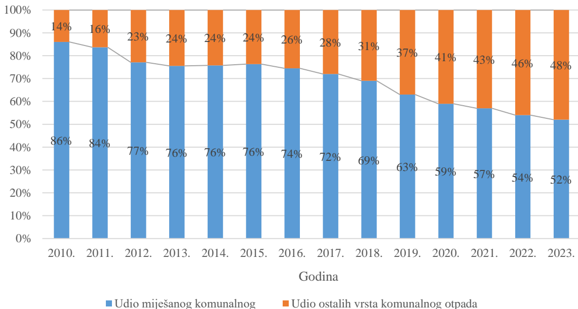
Slika 6. Udio odvojeno sakupljenog komunalnog otpada i miješanog komunalnog otpada u RH, 2010.-2023. godina
