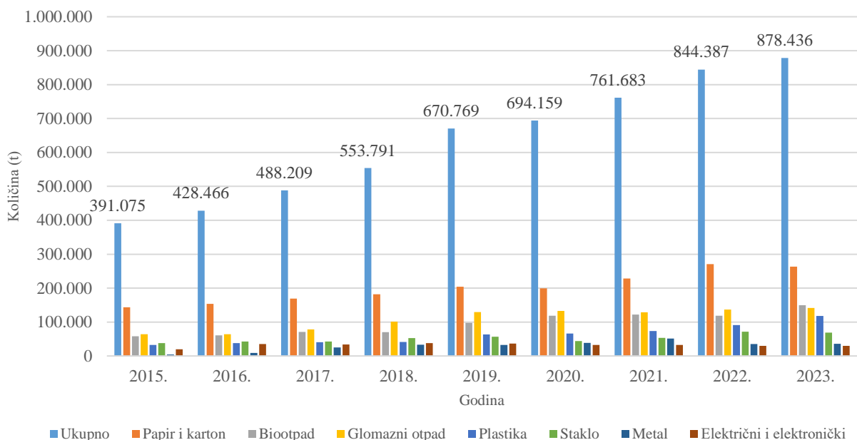
Slika 5. Količine odvojeno sakupljenog komunalnog otpada u RH, 2015.-2023. godina
