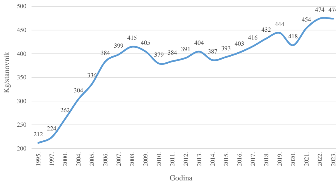
Slika 3. Godišnje količine nastalog komunalnog otpada po stanovniku u RH, 1995.-2023. godina 7
