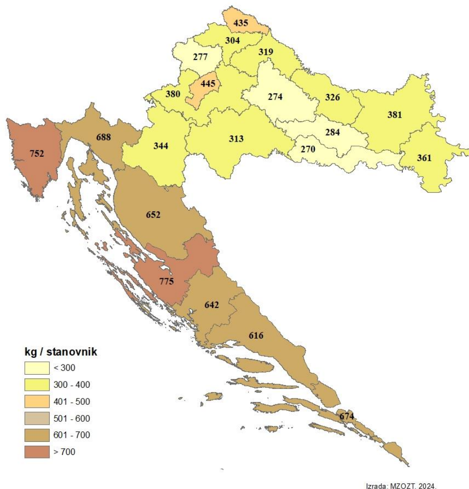
Slika 15. Količine nastalog komunalnog otpada po stanovniku u 2023. godini po županijama
