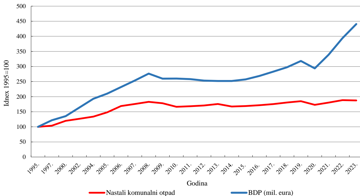
Slika 4. Razdvajanje veze između stvaranja komunalnog otpada i gospodarskog razvoja, 1995. do 2023. godina
