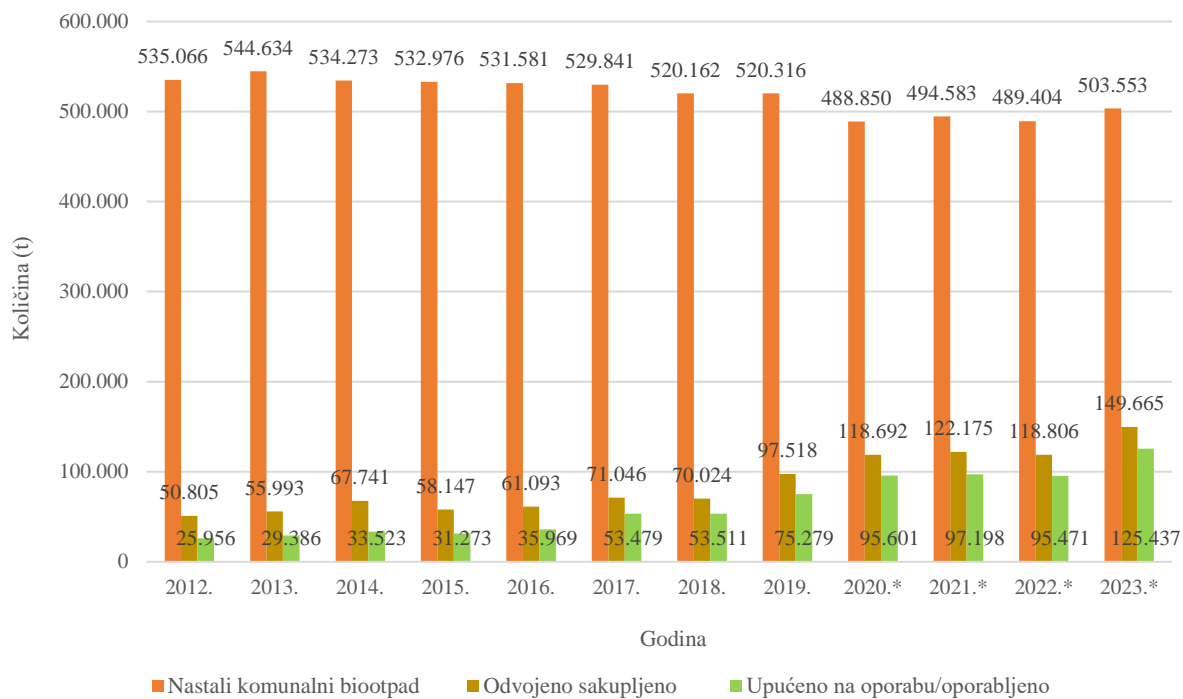
Slika 13. Nastali biootpad iz komunalnog otpada i gospodarenje s istim, 2012.-2023. godina
