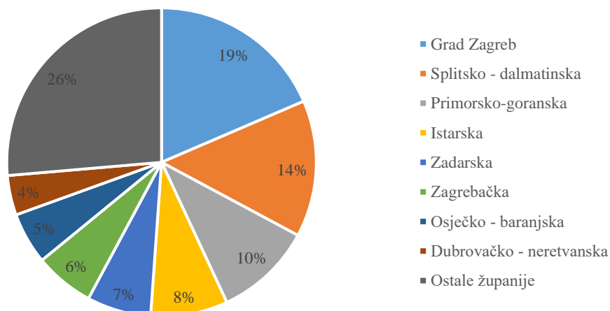
Slika 16. Udjeli pojedinih županija u ukupno sakupljenom komunalnom otpadu u okviru javne usluge u 2023. godini
