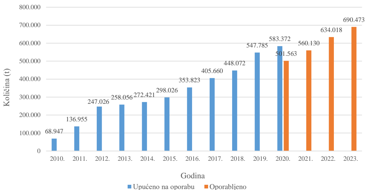
Slika 7. Količine komunalnog otpada upućenog na uporabu / oporabljeno u RH u razdoblju od 2010.-2023. godine
