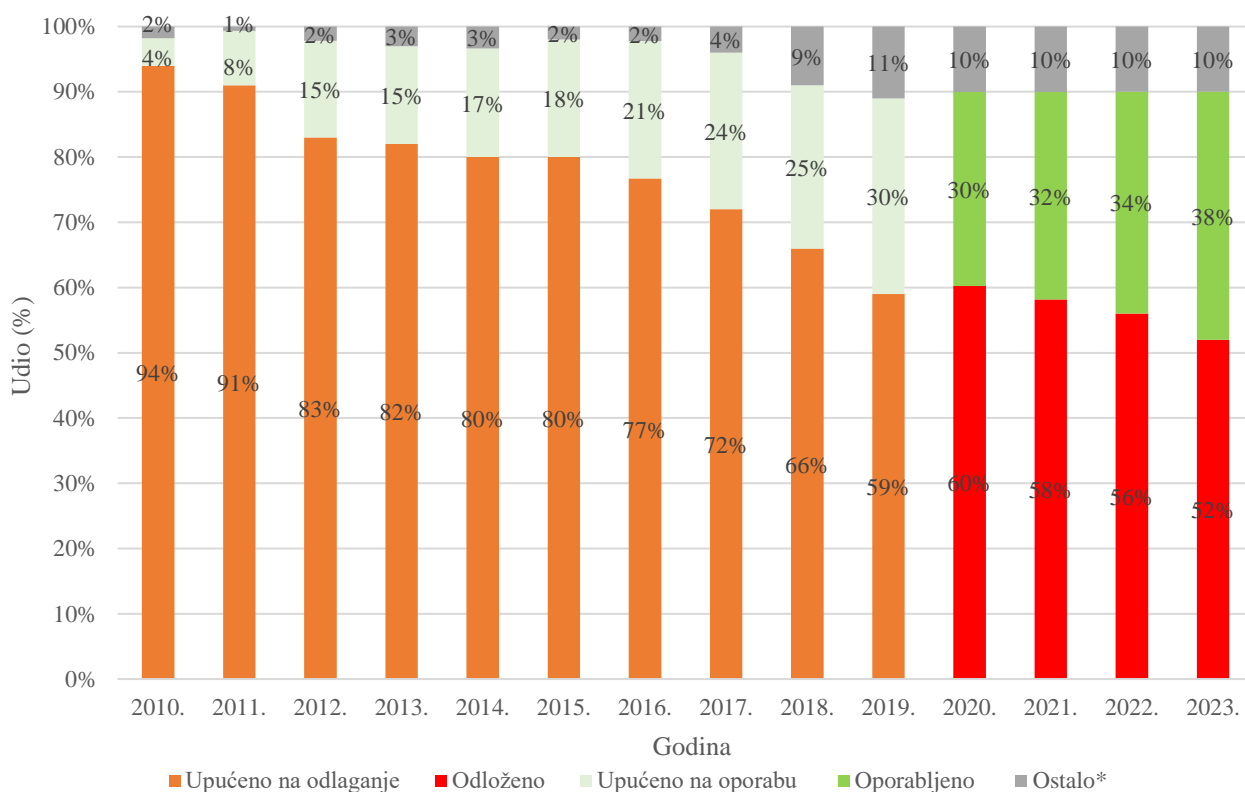
Slika 9. Udio komunalnog otpada RH po postupcima obrade, 2010.- 2023. godina
