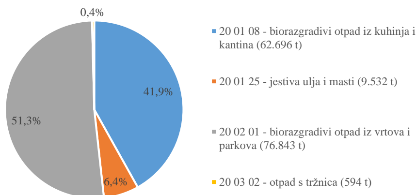
Slika 24. Količine i udjeli pojedinih vrsta komunalnog biootpada u odvojeno sakupljenim količinama u 2023. godini
