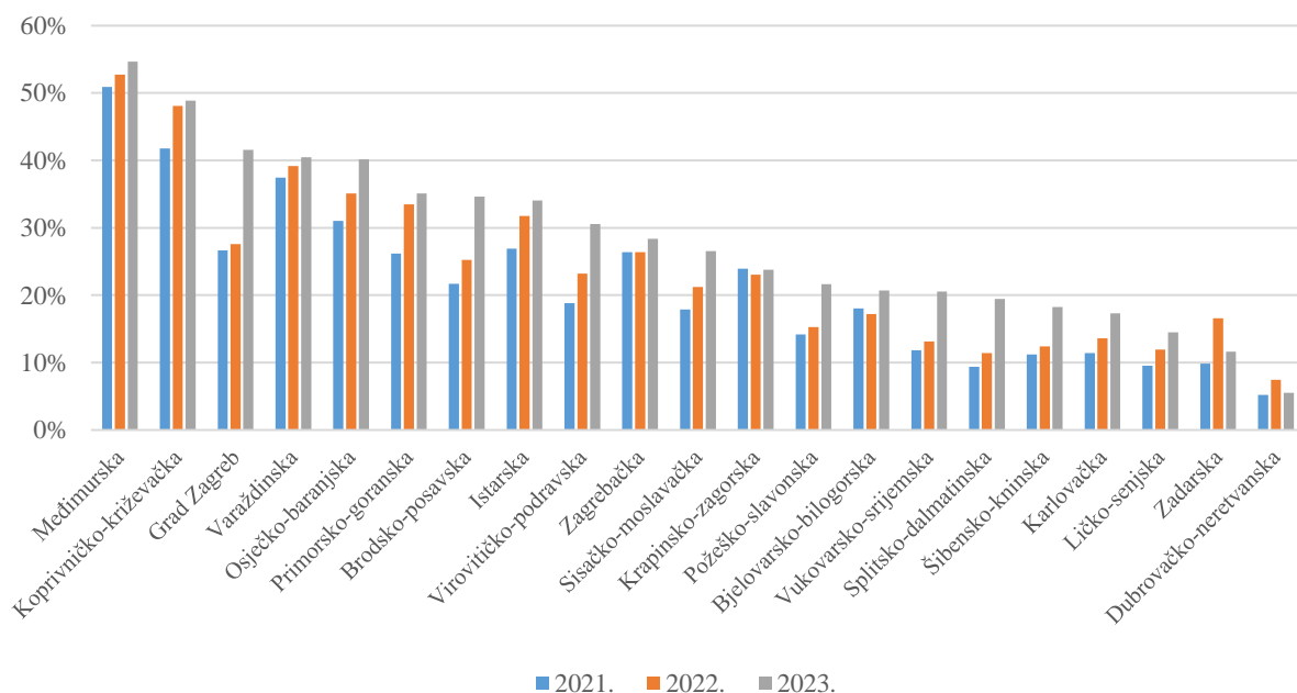
Slika 17. Stopa odvojenog sakupljanja u okviru javne usluge u razdoblju od 2021. do 2023. godine, po županijama
