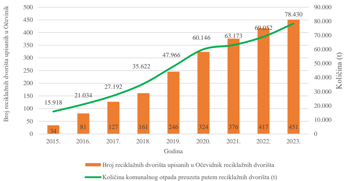
Slika 19. Broj reciklažnih dvorišta upisanih u Očevnik reciklažnih dvorišta i količine komunalnog otpada sakupljene putem reciklažnih dvorišta u razdoblju od 2015. do 2023. godine
