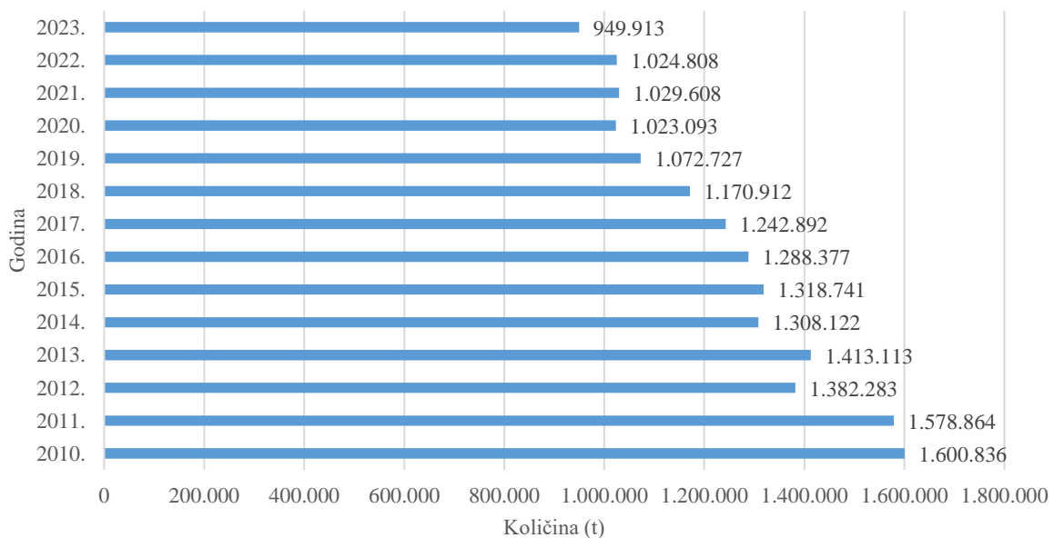
Slika 10. Količine odloženog komunalnog otpada, 2010.-2023. godina
