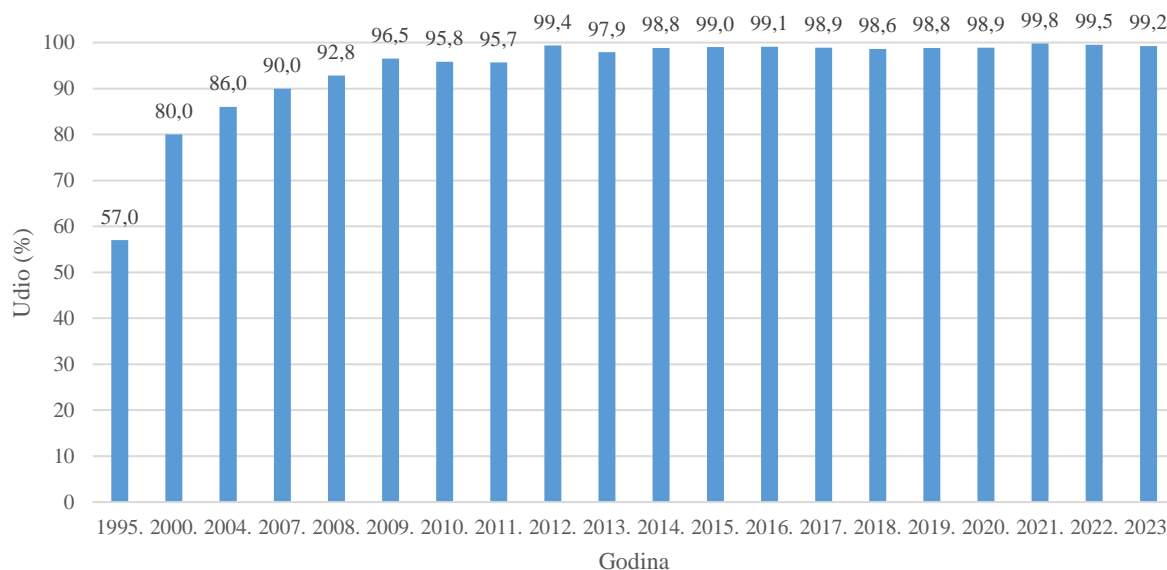
Slika 1. Obuhvat stanovništva organiziranim sakupljanjem komunalnog otpada u RH u razdoblju od 1995. do 2023. godine
