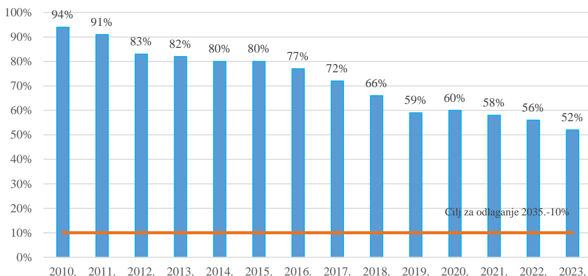
Slika 11. Udio odlaganja komunalnog otpada u razdoblju od 2010. do 2023. godine u odnosu na propisani cilj za 2035. godinu
