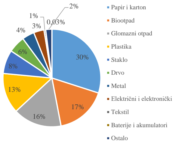
Slika 18. Odvojeno sakupljeni komunalni otpad u 2023. godini, po vrstama
