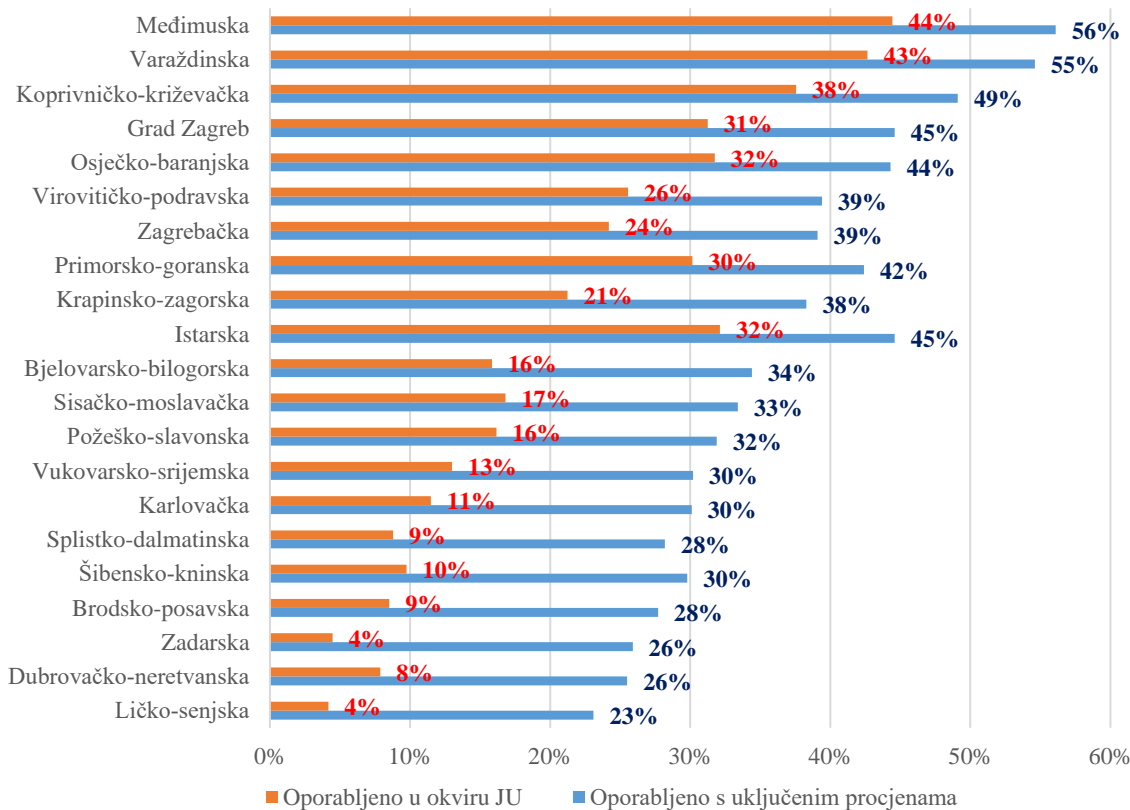
Slika 21. Stopa oporabe komunalnog otpada u 2023. godini po županijama, u okviru javne usluge i s uključenim procjenama
