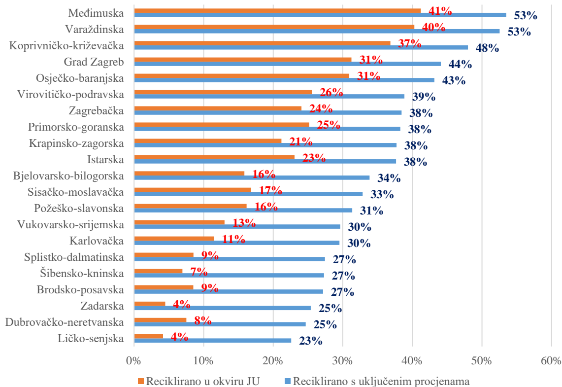
Slika 20. Stopa recikliranja komunalnog otpada u 2023. godini po županijama, u okviru javne usluge i s uključenim procjenama
