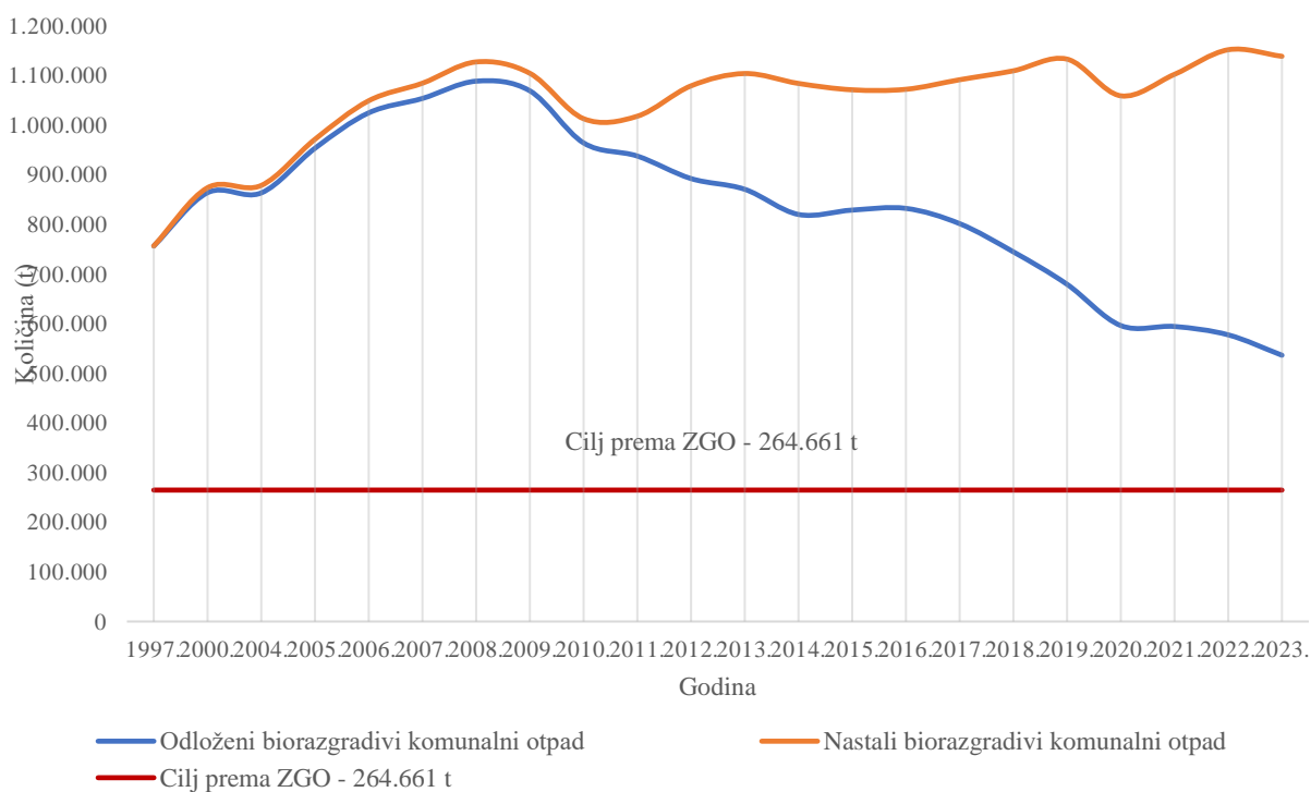
Slika 12. Nastali i odloženi biorazgradivi komunalni otpad za razdoblje od 1997. do 2023. godine u odnosu na ciljanu količinu propisanu ZGO-om
