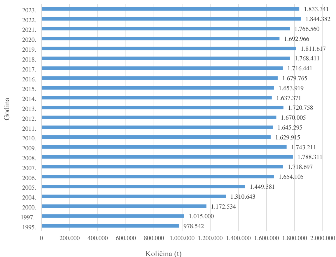
Slika 2. Količine ukupno nastalog komunalnog otpada u RH, 1995.-2023. godina
