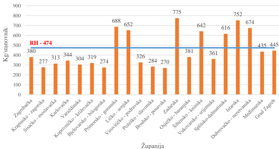
Slika 14. Odnos količine nastalog komunalnog otpada po stanovniku po županijama i količine nastalog komunalnog otpada po stanovniku za RH u 2023. godini
