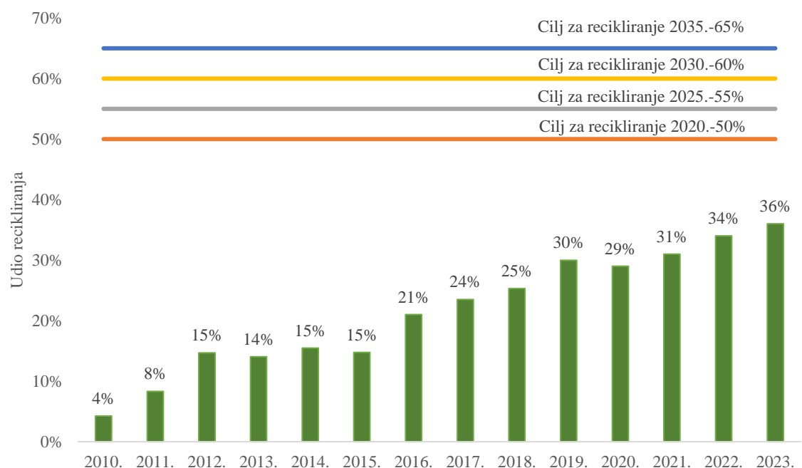
Slika 8. Udio recikliranja u RH u razdoblju od 2010. do 2023. godine u odnosu na propisane ciljeve
